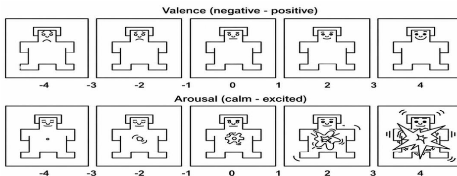
Fig. 3 SAM scale [28]
