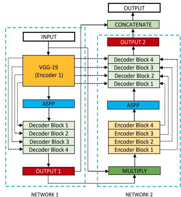
Fig. 4 DoubleUnet[16]
