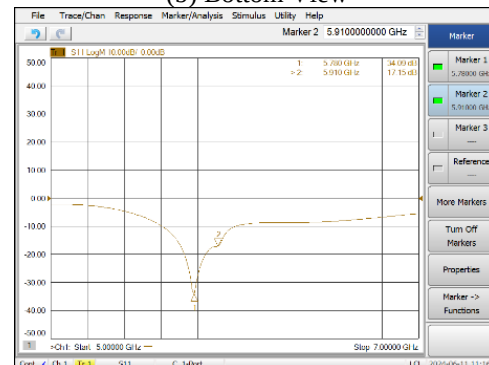
(d) Measured Return Loss
